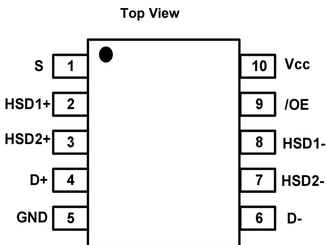
Fig.5-2.GT4222: MA (MSOP10) Package
