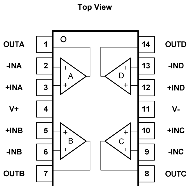
Fig.5-6. GT8114: TD (TSSOP14) Package
